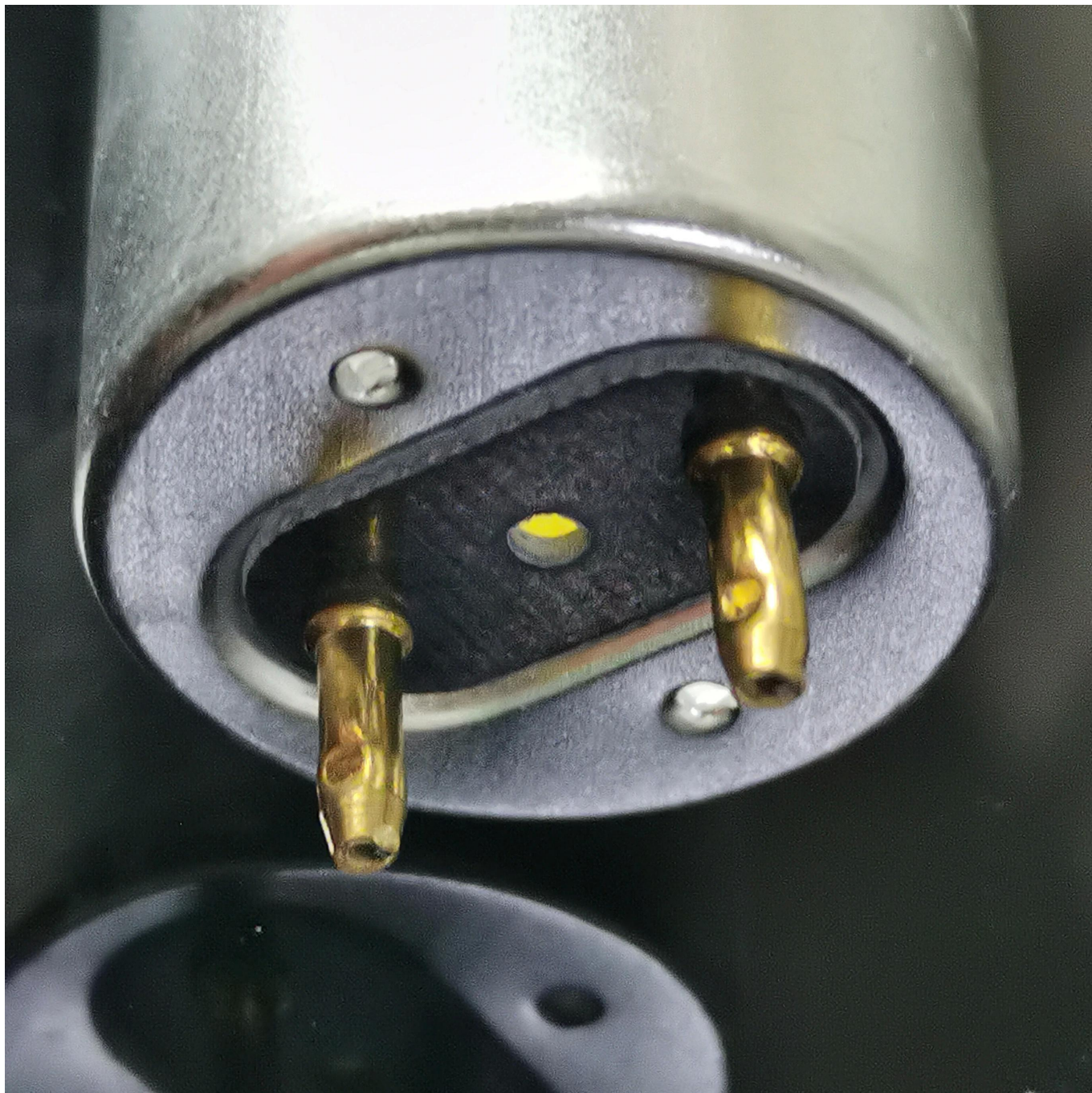
Lámpara esterilizadora UVC del fabricante chino Se utilizan ampliamente en sistemas de desinfección de aire, sistemas de tratamiento de agua, industria de pintura, industria de impresión, etc.
