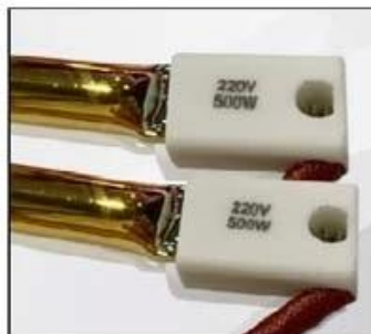
All Gold IR lamp
